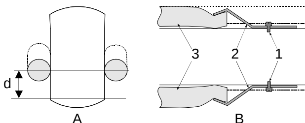
Abbildung 20: Autogrip-Welle
