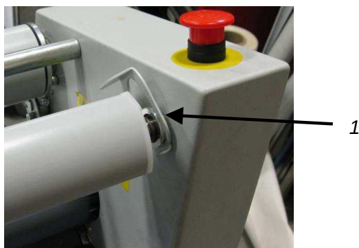
Figure 11 : Dispositif de verrouillage en haut
