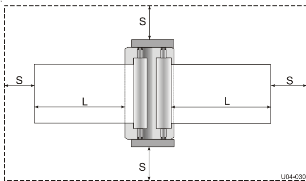
Abbildung 4: Arbeitsplatz
