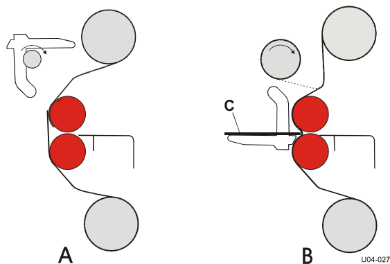
Figure 18 : Amorçage de la partie inférieure
