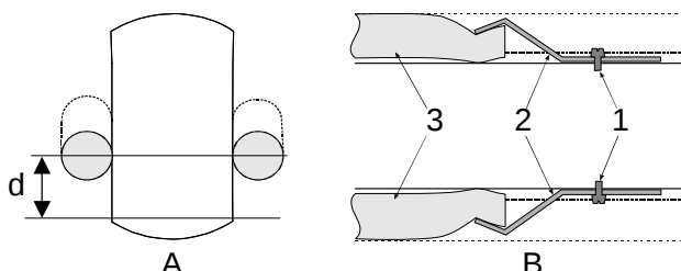
Figure 20 : Mandrin antidérapant
